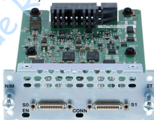
Figura 17. Módulo NIM-2T
