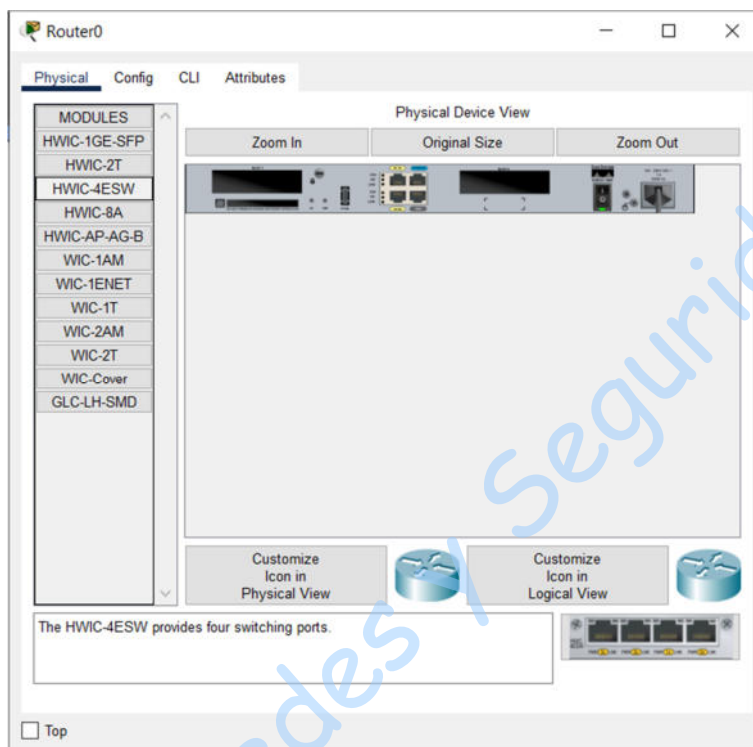
Figura No. 8. Descripción e imagen del módulo HWIC-4ESW.
