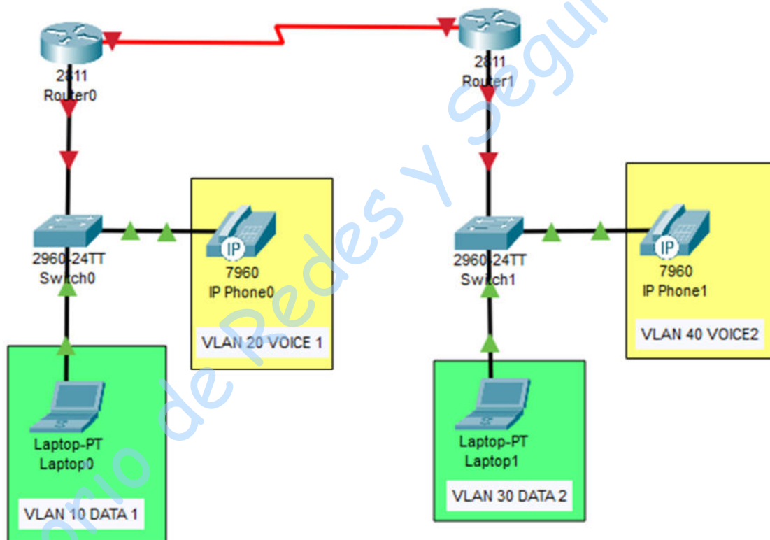
Figura No. 4 Topología de Red.
