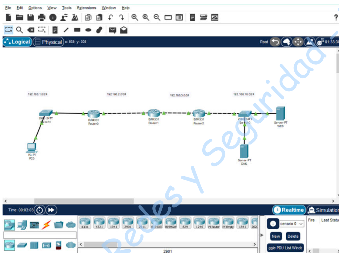
Figura No. 3. Topología.
