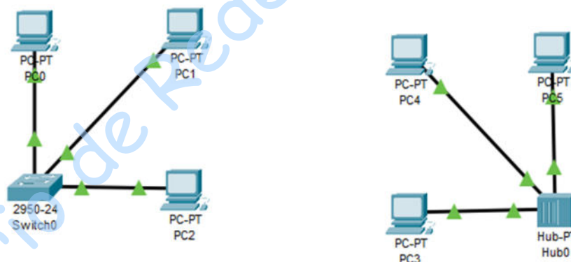
Figura No. 15. Topología de red.
