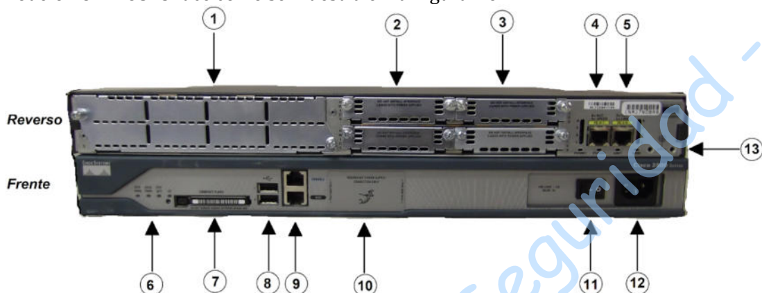
Figura 2. Modelo 2811 IOS15.
