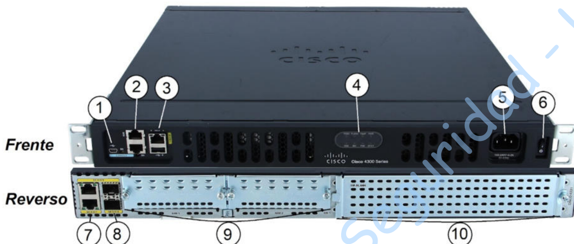
Figura No. 3. Modelo ISR4331.
