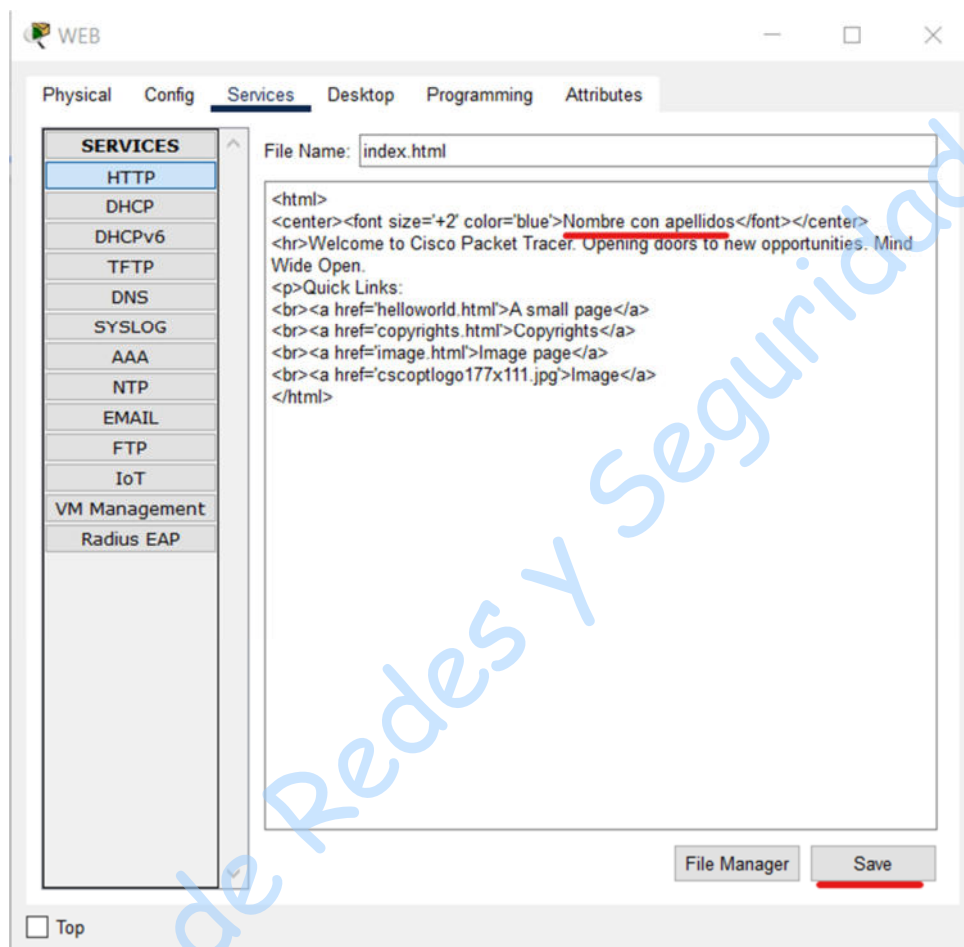
Figura No. 8. Archivo index.html editado.
