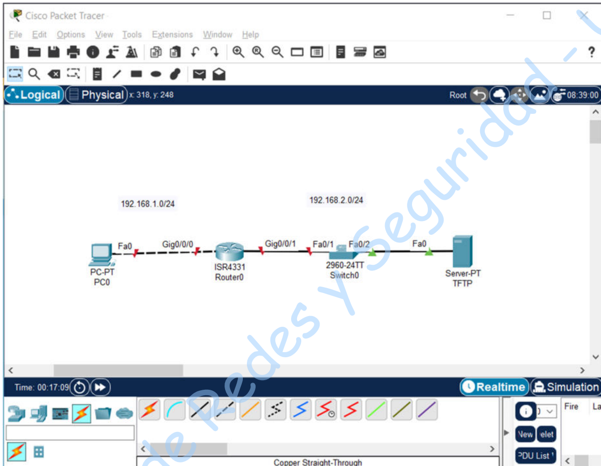
Figura No. 2. Topología para TFTP
