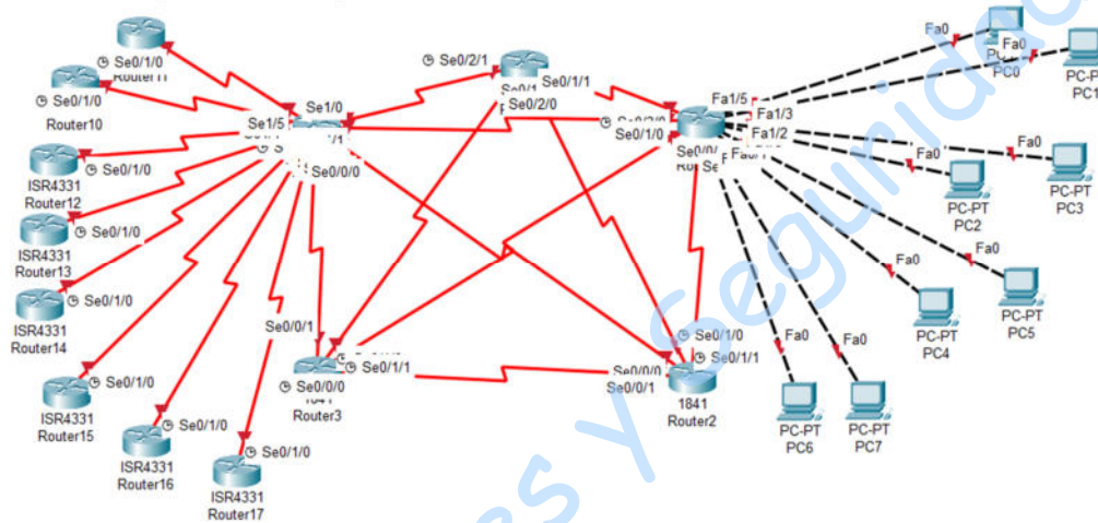
Figura 21. Topología 1 para armar.
