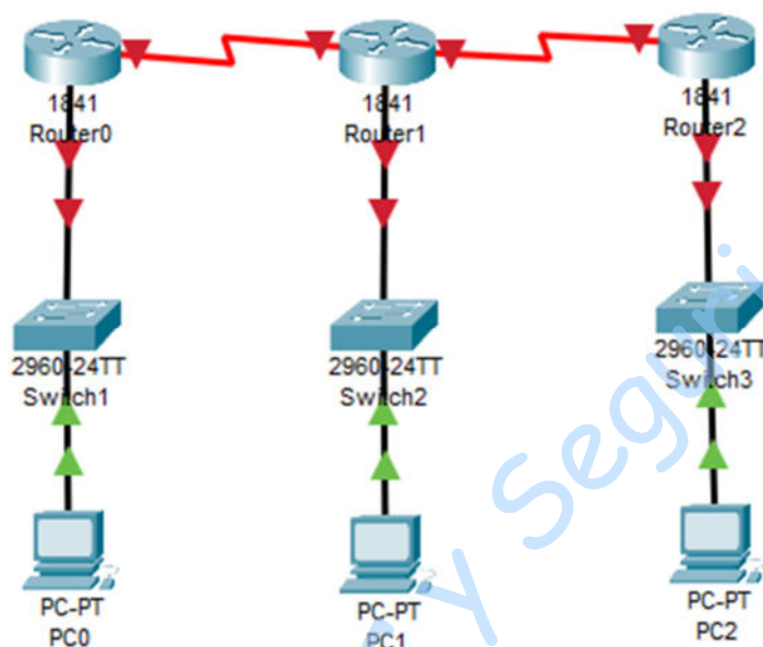
Figura No. 5. Conexión de los routers
