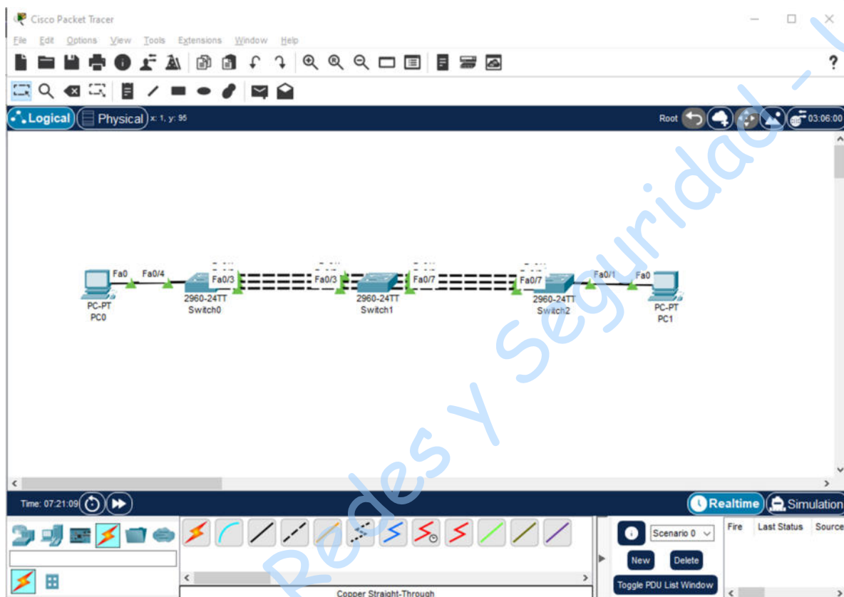
Figura No. 10. Topología para armar
