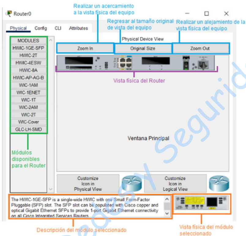
Figura No. 7. Módulos disponibles para el modelo 1841.
