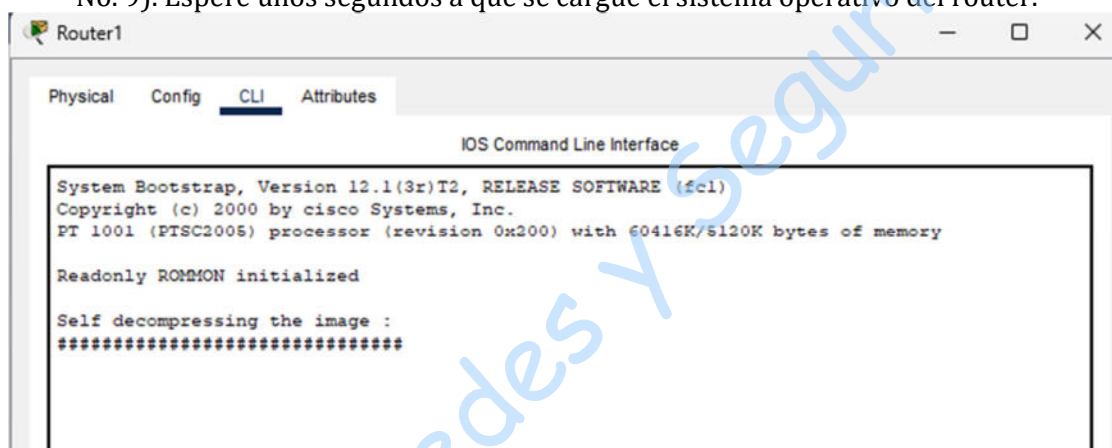
Figura No. 9. Interfaz de consola del router.
