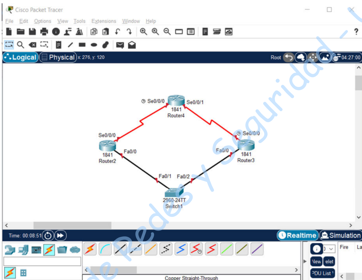
Figura No. 3. Topología para configurar HSRP
