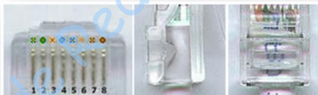
Figura No. 5. Alambres y forro en el lugar adecuado dentro del conector
