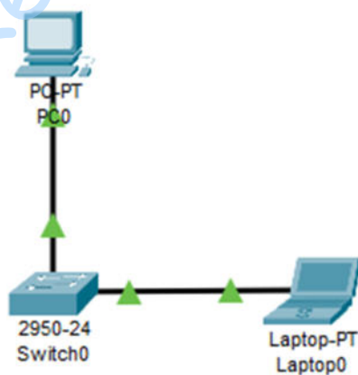
Figura No. 3. Topología básica
