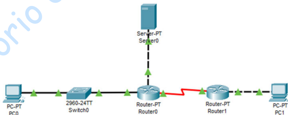
Figura No. 10 Topología de red final
