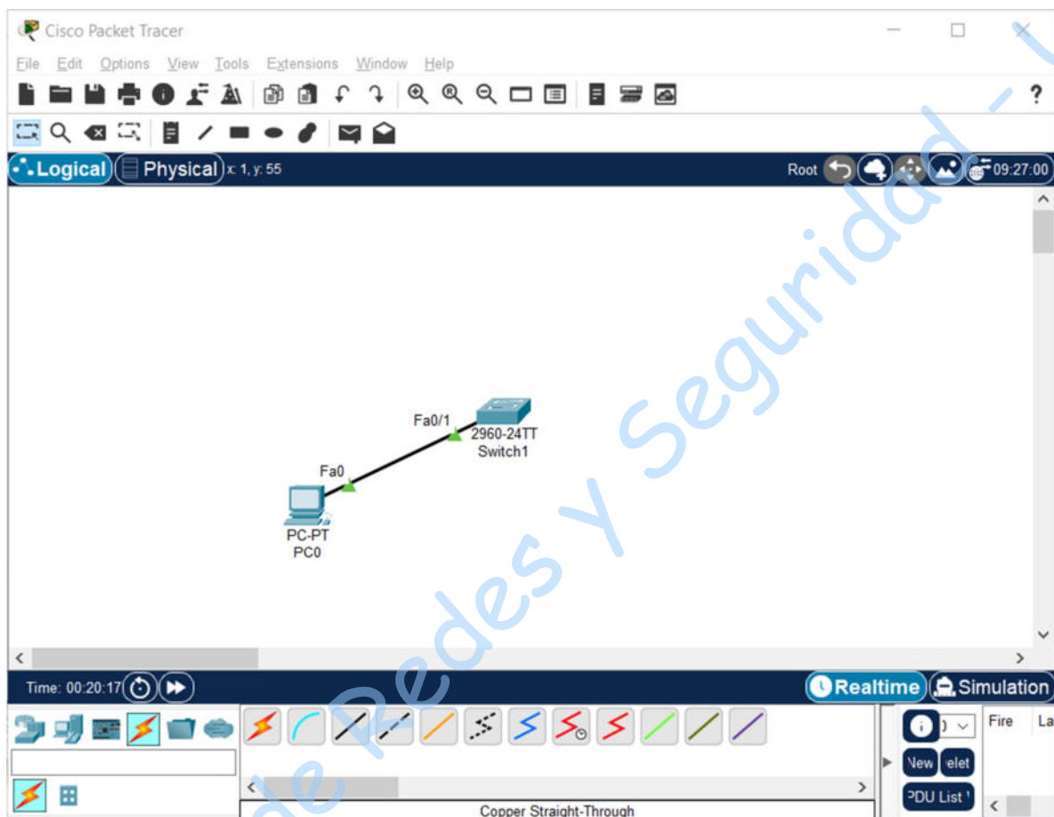
Figura No. 11. Topología configuración port security
