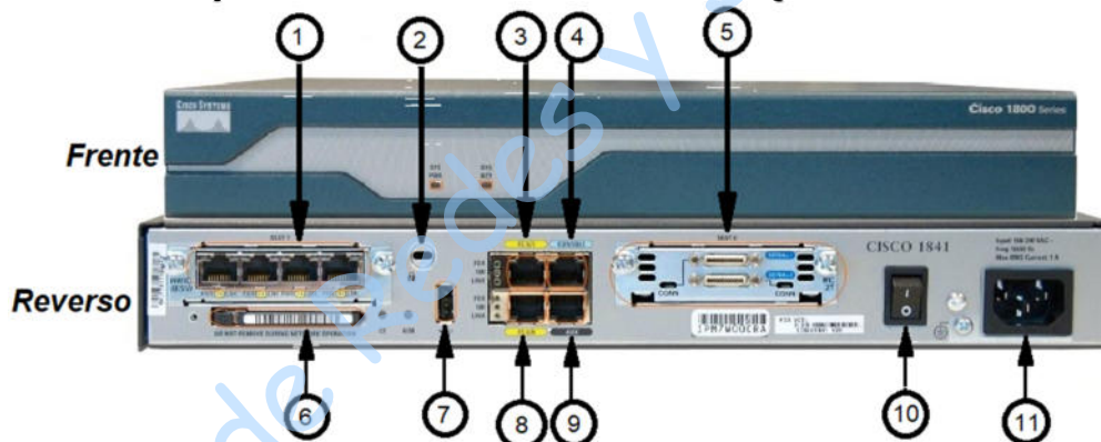
Figura No. 1. Modelo 1841.
