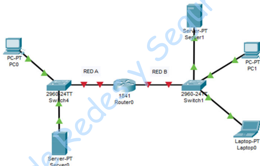
Figura No. 3. Topología básica
