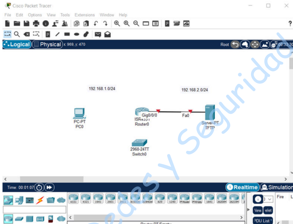
Figura No. 8. Conexión necesaria para eliminación y recuperación del SO de un Router
