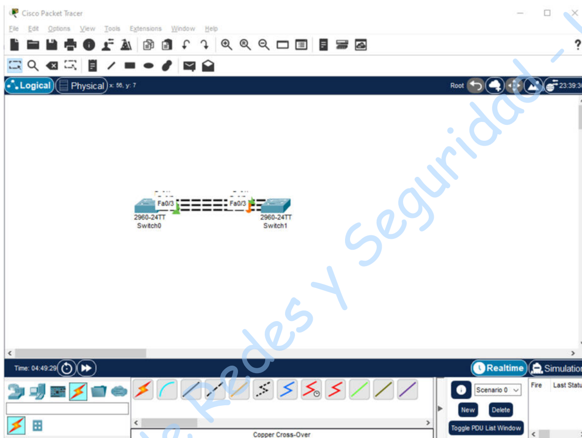
Figura No. 3. Switch 0 y 1 conectados
