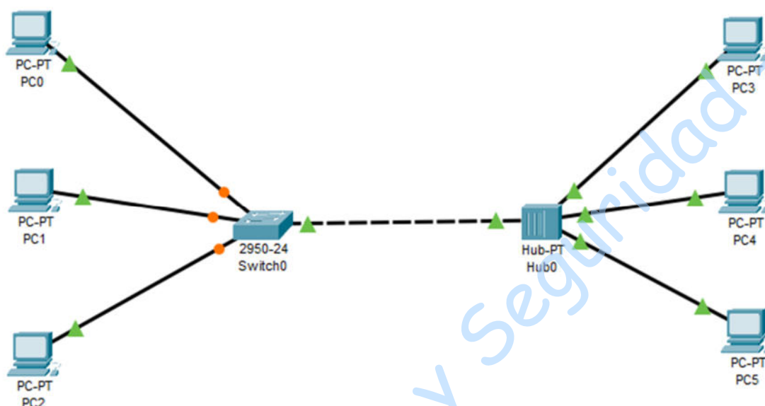
Figura No. 3 Creando la topología en Cisco Packet Tracer.
