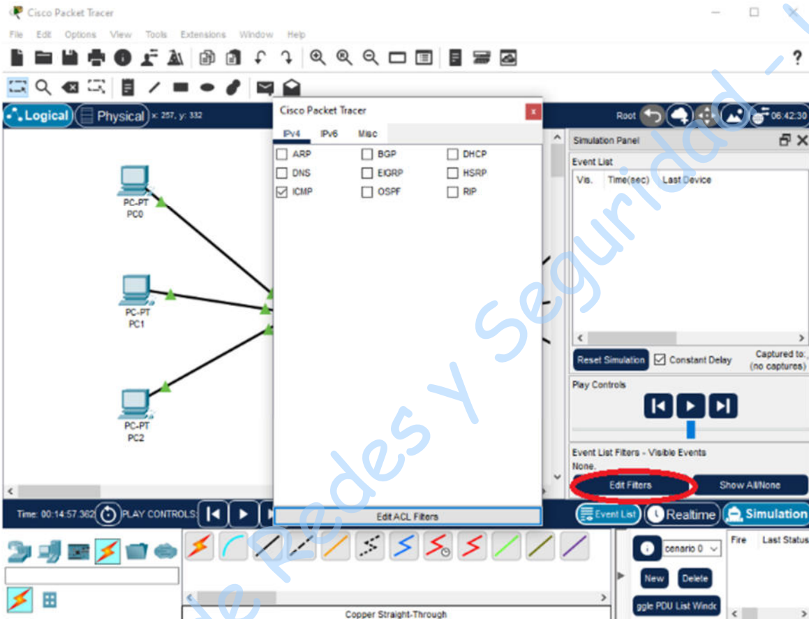
Figura No. 8 Simulación de Packet Tracer en curso.
