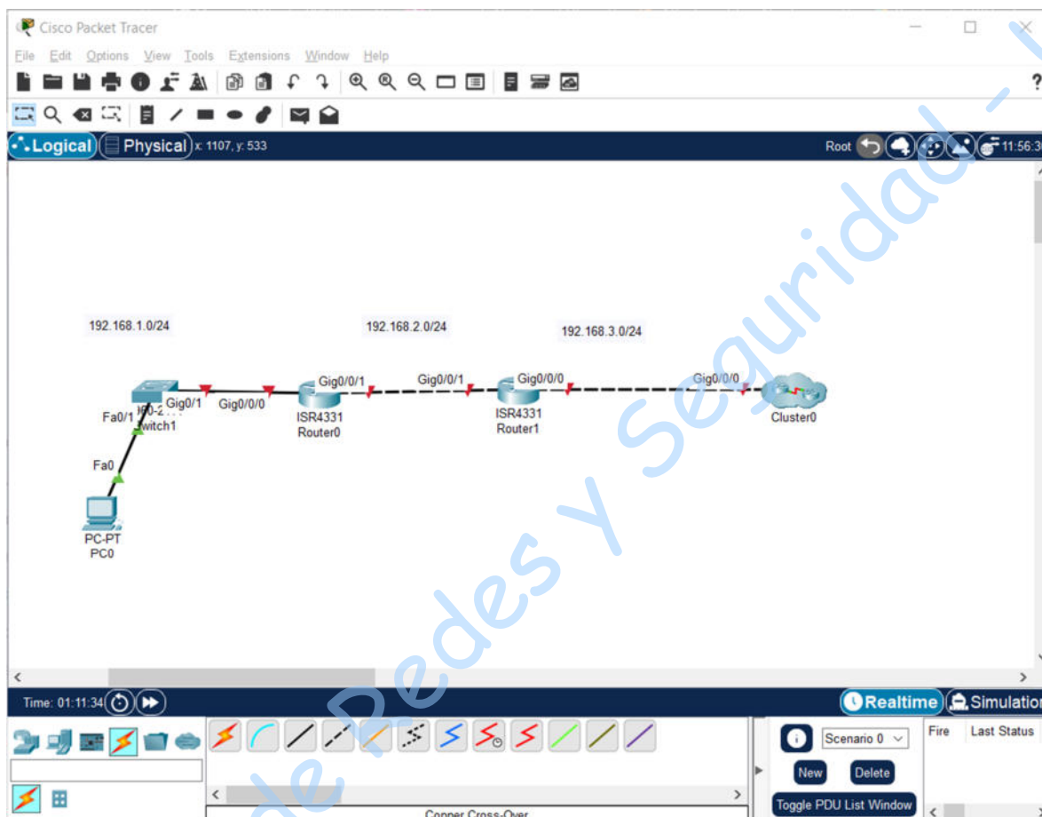
Figura No. 4. Topología con el clúster hecho.
